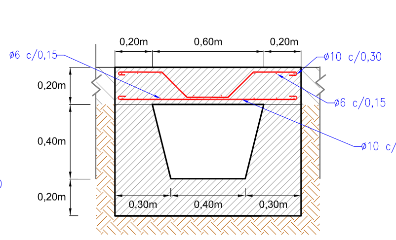
MURO DE SOSTENIMIENTO CON CUNETAS TRAPEZIAL Secc. 4
