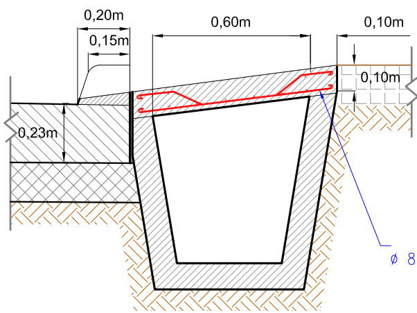
MURO DE SOSTENIMIENTO CON CUNETAS TRAPEZIAL Secc. 3
