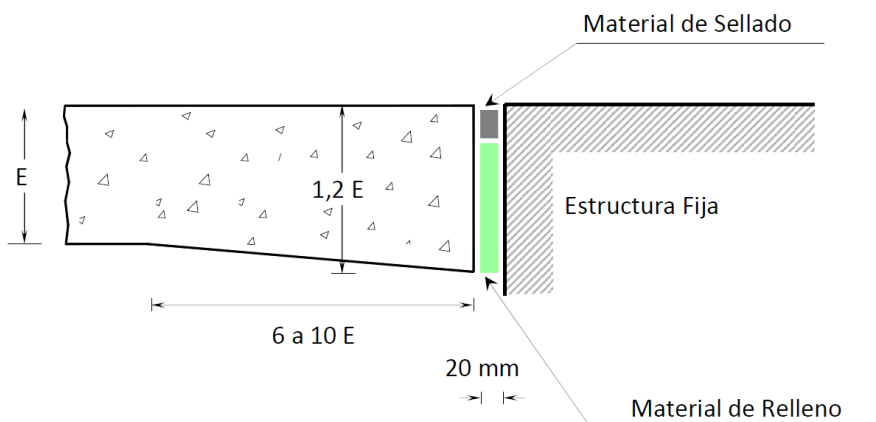
Detalle de junta de aislación con sobreespesor de hormigón, contra estructura fija
