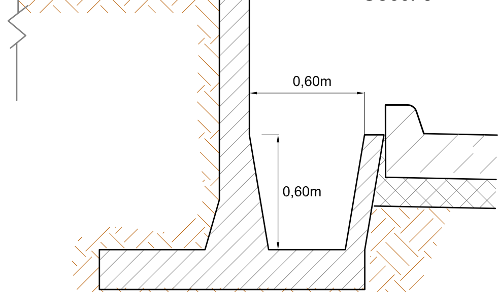
MURO DE SOSTENIMIENTO CON CUNETAS TRAPEZIAL Secc. 3
