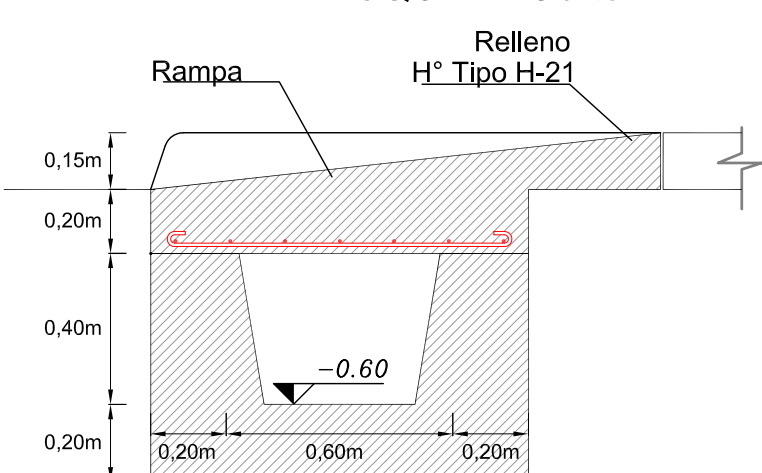
DETALLE DE ESQUINA Corte B-B
