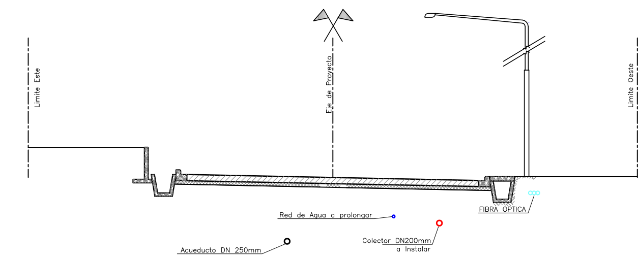
PERFIL TRANSVERSAL ESC 1:125
