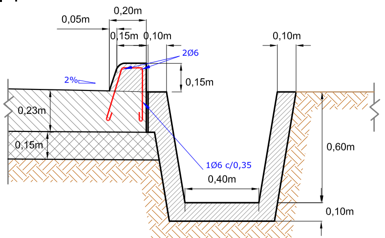
CORDÓN INTEGRAL-CUNETAS TRAPEZIAL Secc. 1
