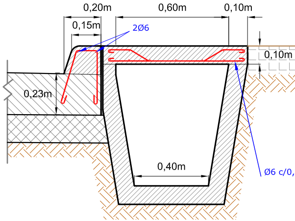
MURO DE SOSTENIMIENTO CON CUNETAS TRAPEZIAL Secc. 4
