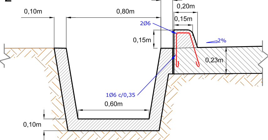
CORDÓN INTEGRAL-CUNETAS TRAPEZIAL Secc. 2
