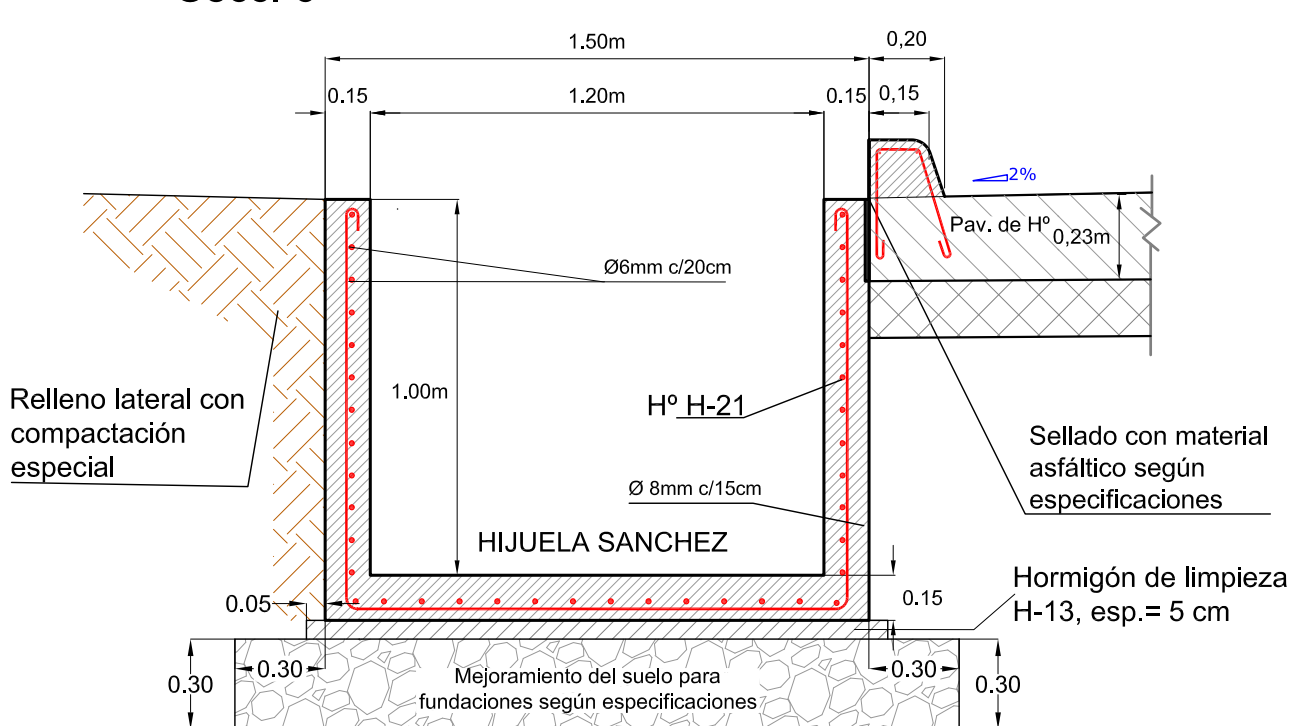
CANAL RECTANGULAR DE HORMIGÓN Y DETALLE DE CORDÓN INTEGRAL Secc. 6
