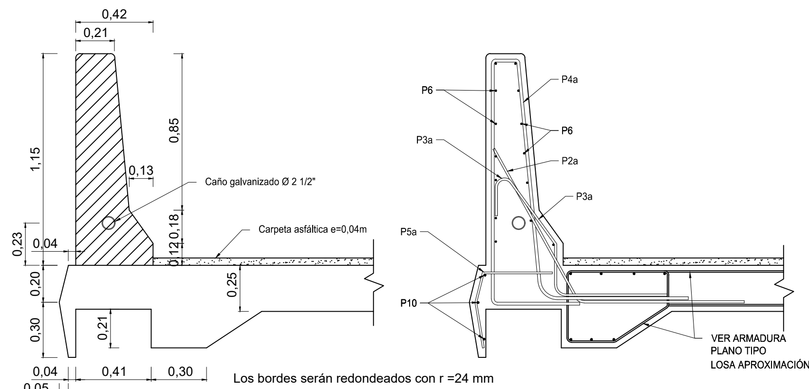
DETALLE EN LOSA DE APROXIMACIÓN Esc. 1:20
