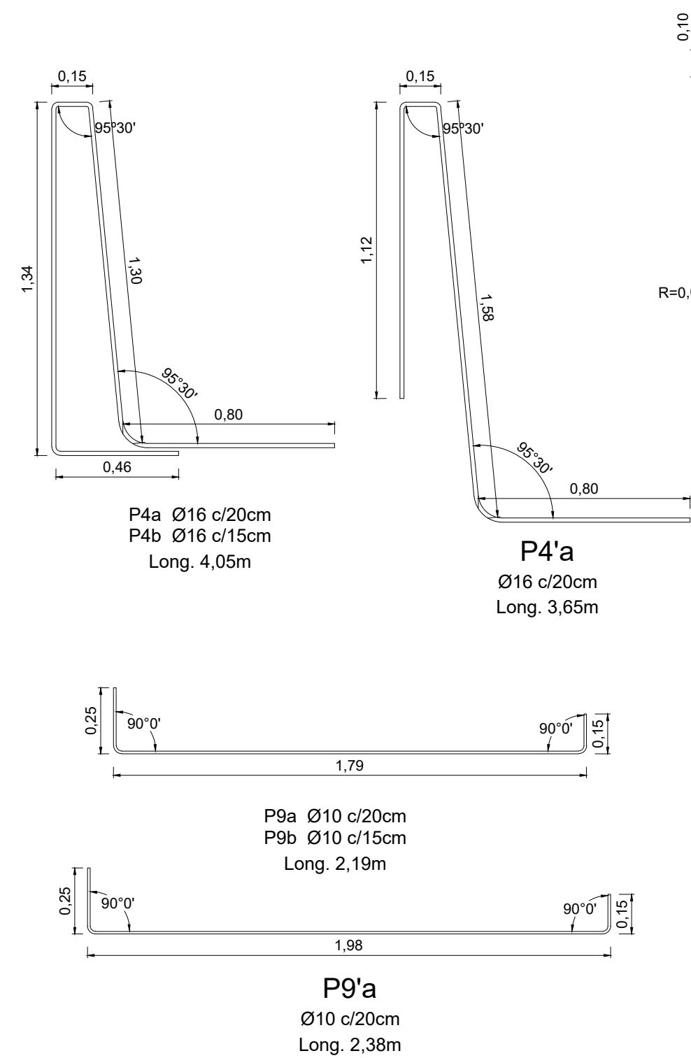
DETALLE ZONA MURO DE ACCESO A PUENTE Esc. 1:20
