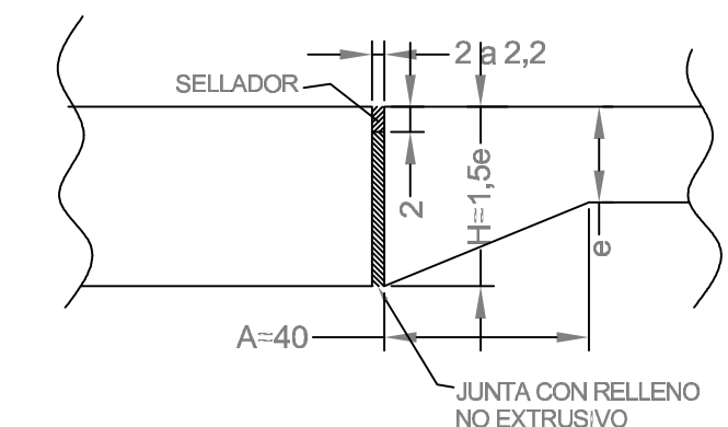
DETALLE JUNTA TIPO C (cm)
