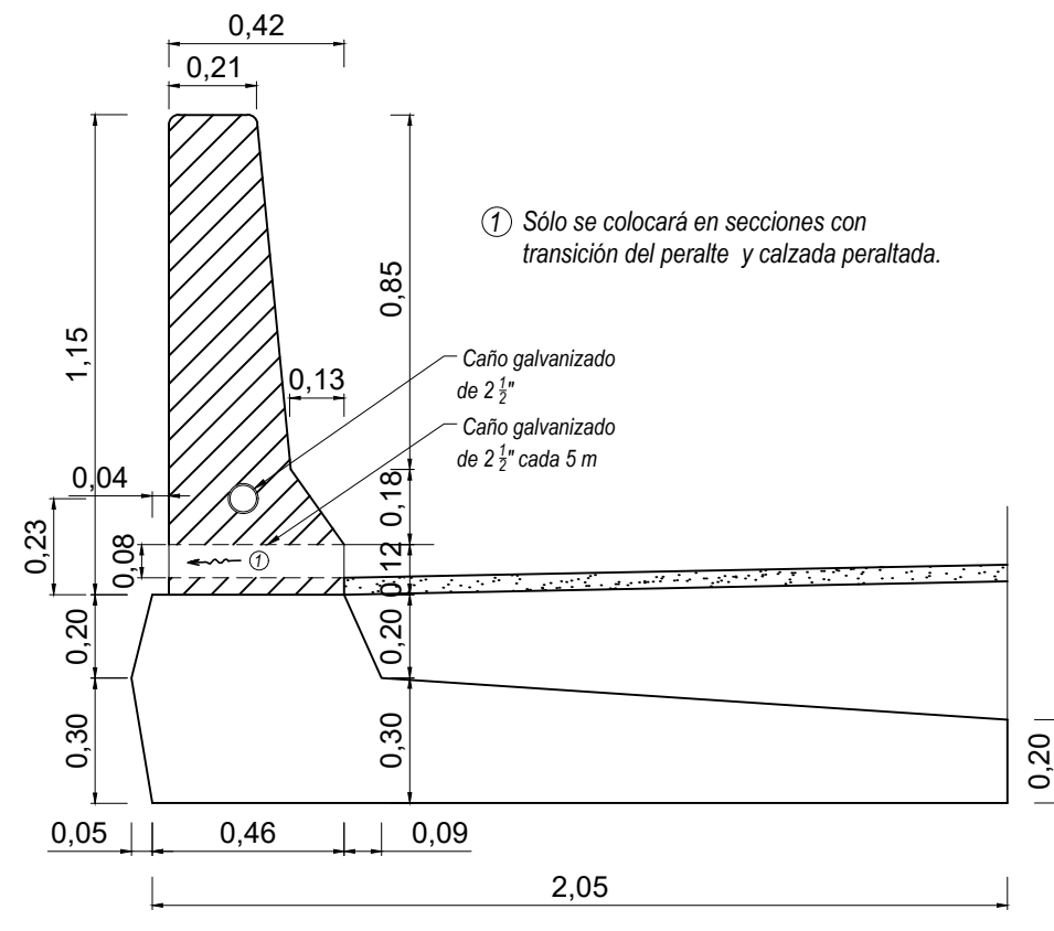
DETALLE ZONA TERRAPLÉN DE ACCESO A PUENTE Esc. 1:20
