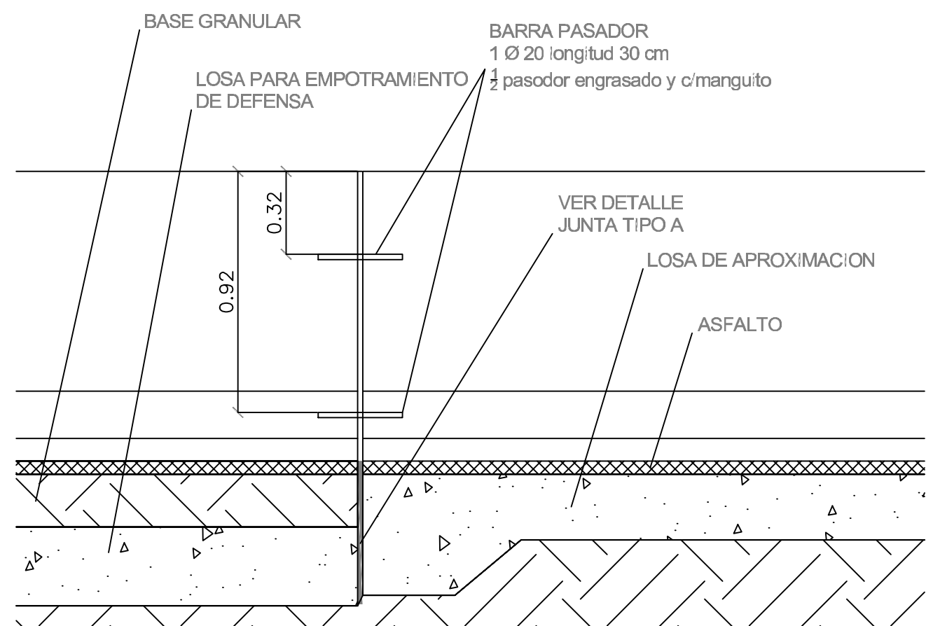
VISTA LATERAL ENCUESTRO LOSA APROXIMACION CON LOSA DE EMPOTRAMIENTO Esc. 1:20
