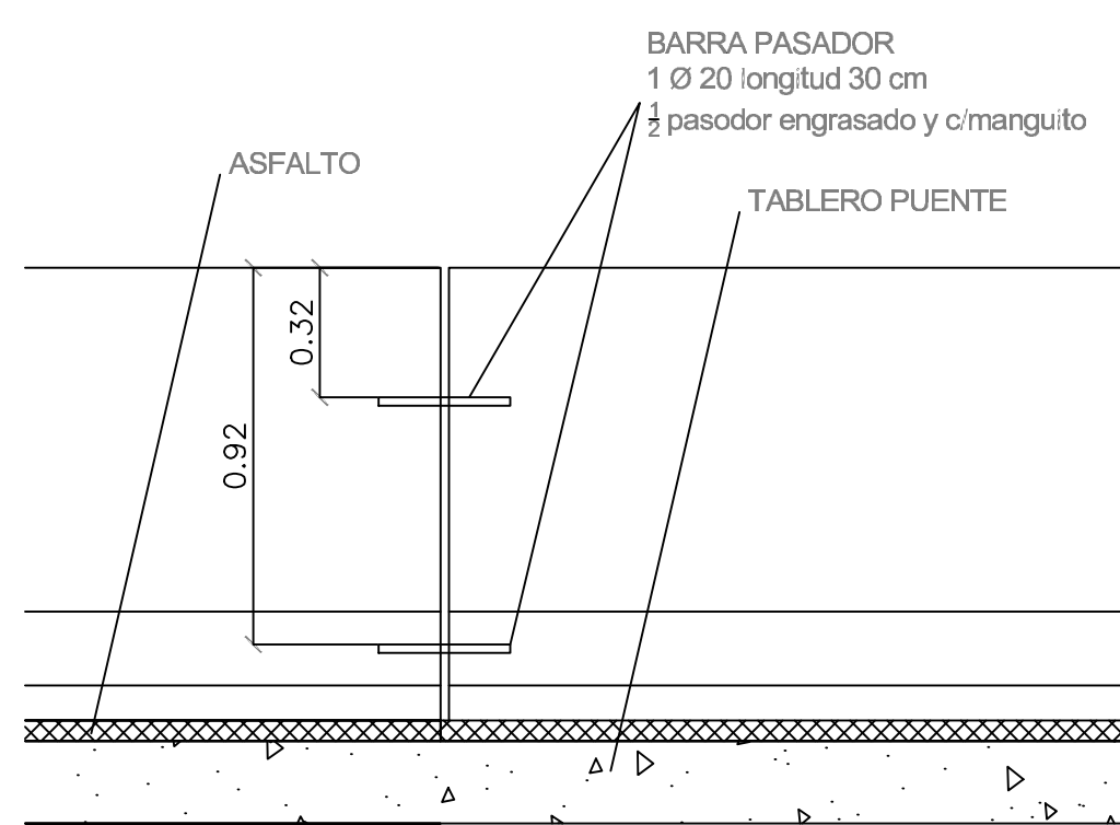
VISTA LATERAL JUNTA EN PUENTE Esc. 1:20
