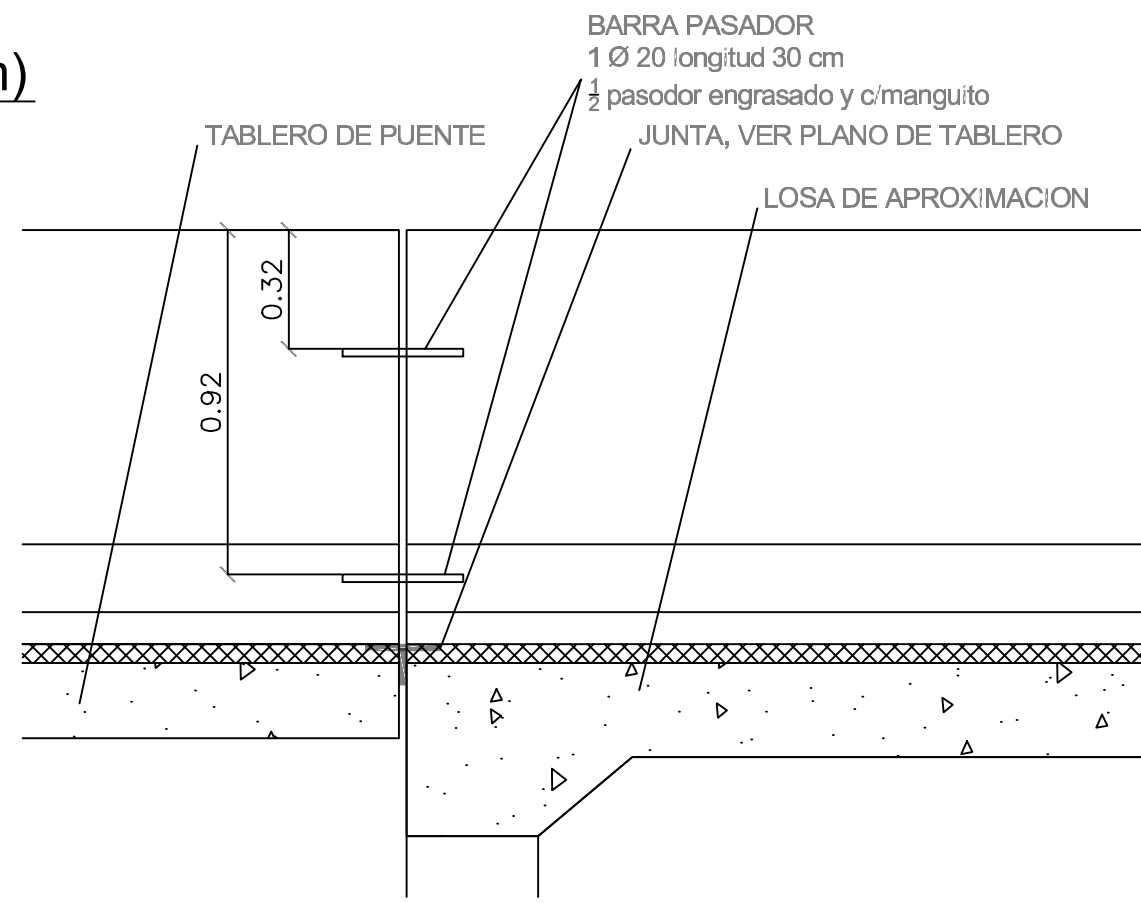
VISTA LATERAL JUNTA EN PUENTE Esc. 1:20
