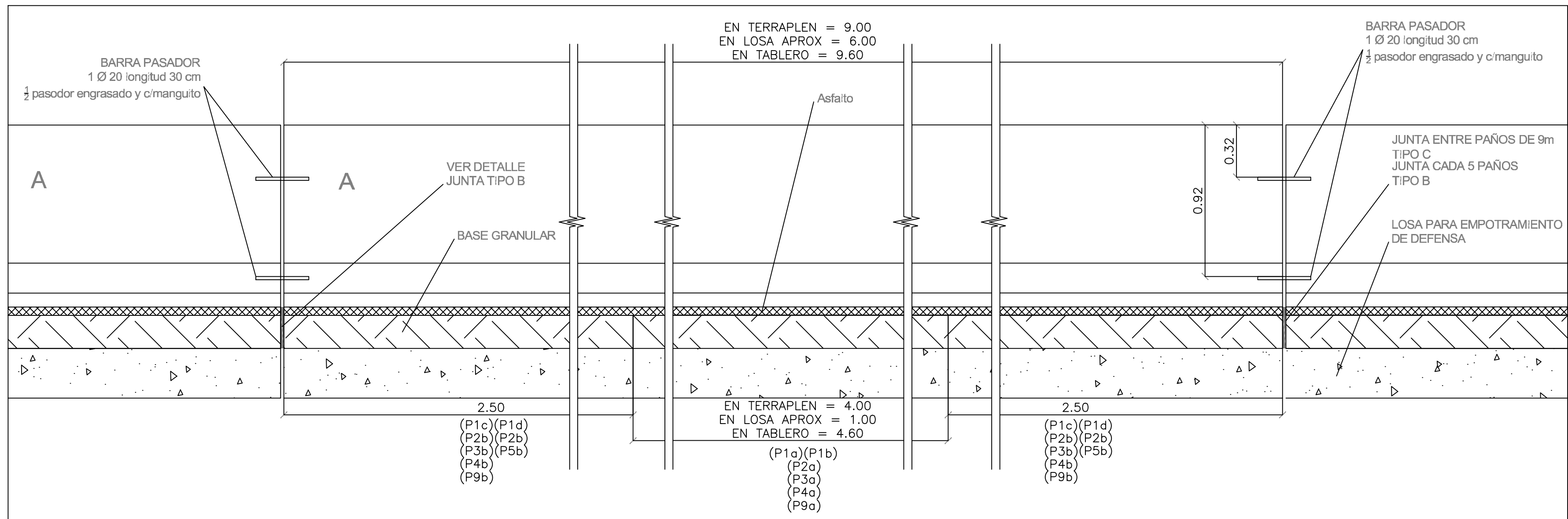
VISTA LATERAL CON DETALLE DE ARMADOS Esc. 1:20
