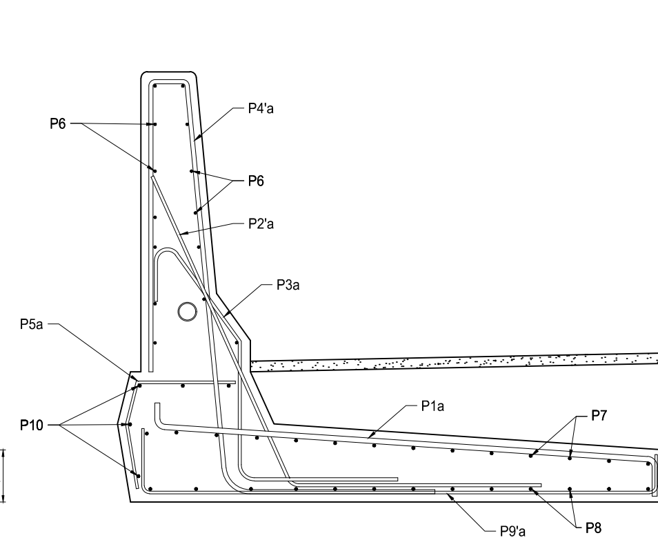
DETALLE ZONA TERRAPLÉN DE ACCESO A PUENTE Esc. 1:20
