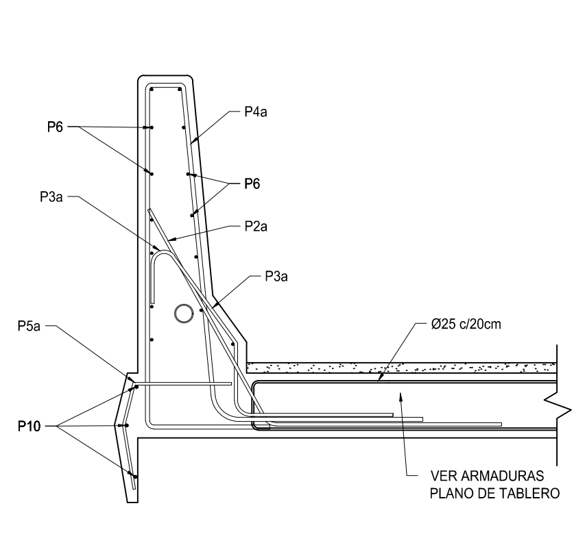
DETALLE EN TABLERO DE PUENTE Esc. 1:20
