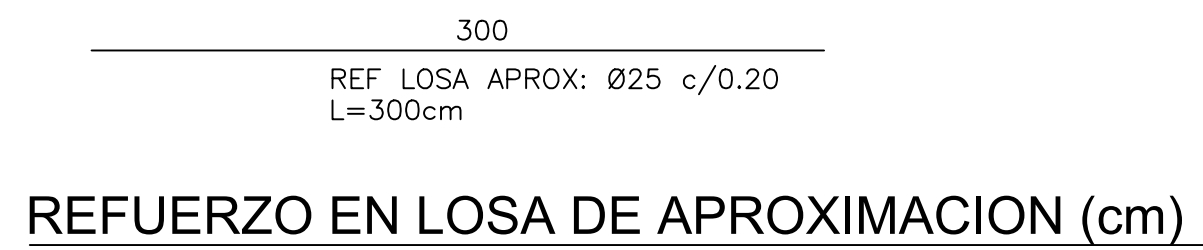
REFUERZO EN LOSA DE APROXIMACION (cm)
