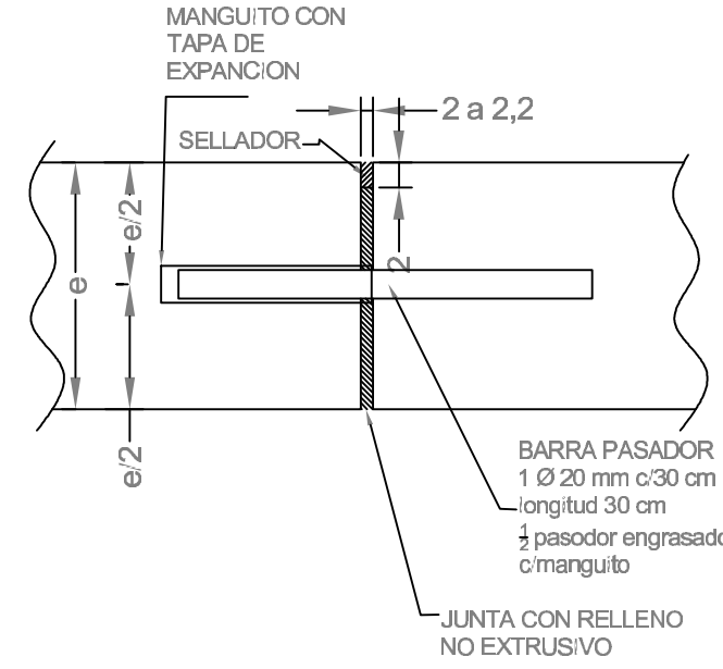
DETALLE JUNTA TIPO C (cm)
