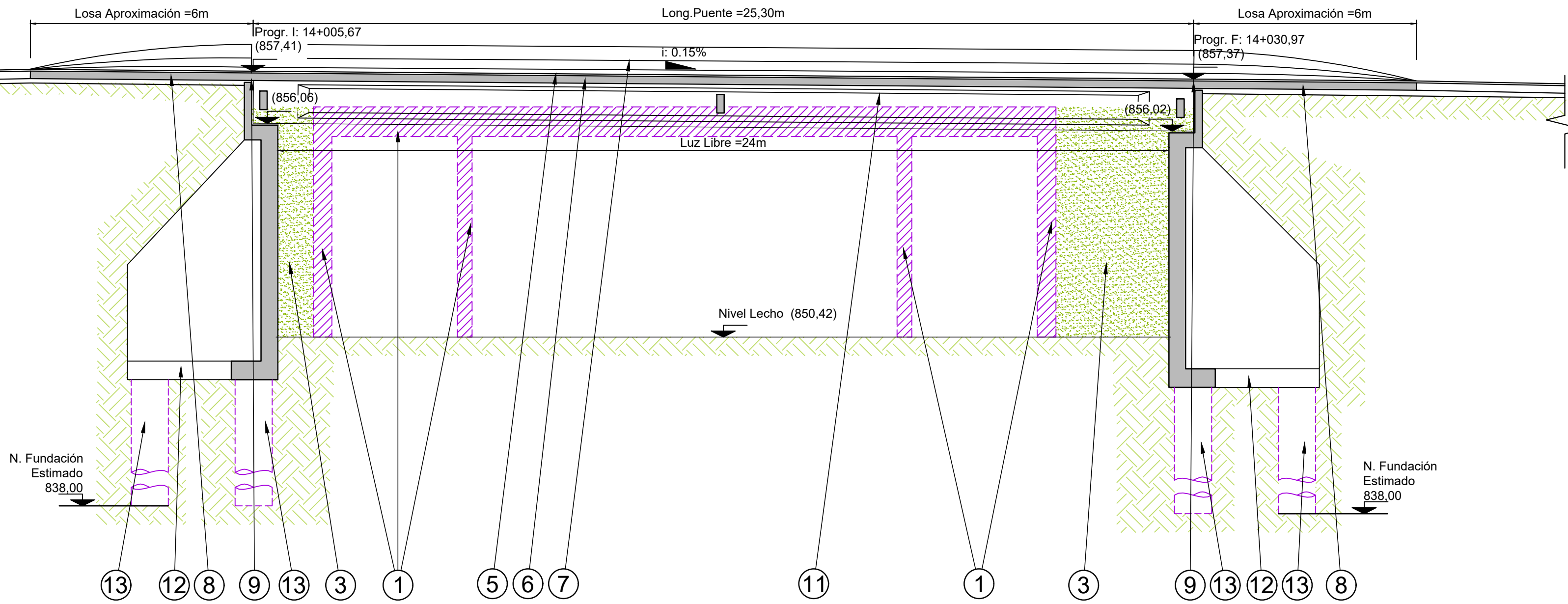
CORTE 1B - 1B Esc. 1:100
