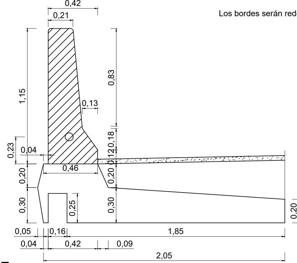
DETALLE ZONA MURO DE ACCESO A PUENTE Esc. 1:20
